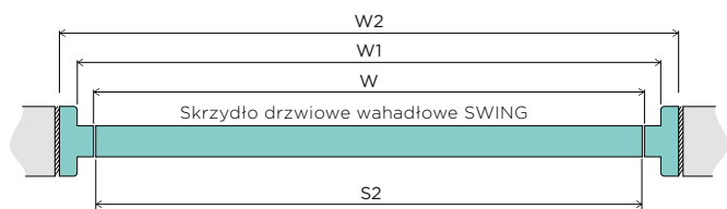
Ościeżnica drzwiowa do drzwi wahadłowych SWING
